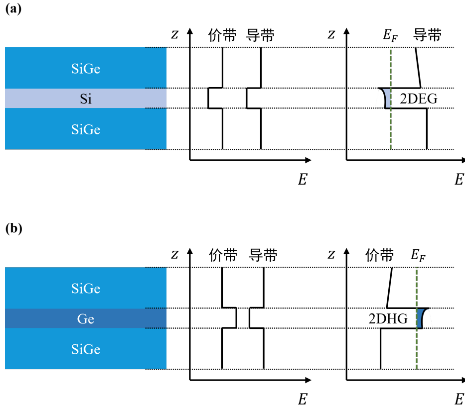
图 1.1 硅锗异质结中的载流子
