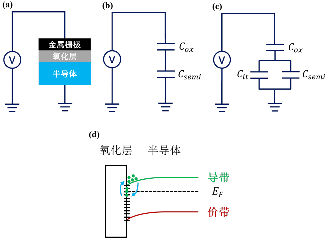
图 2.3 电容-电压法提取界面态示意图
