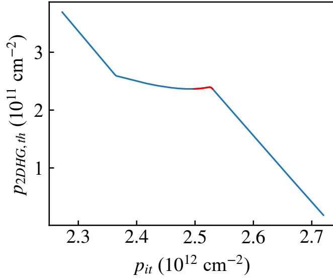
图 4.4 逆向 S-P 计算敏感性分析
