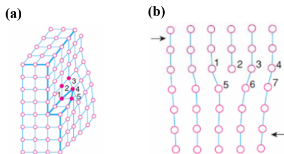
图 1.3 位错滑移示意图
